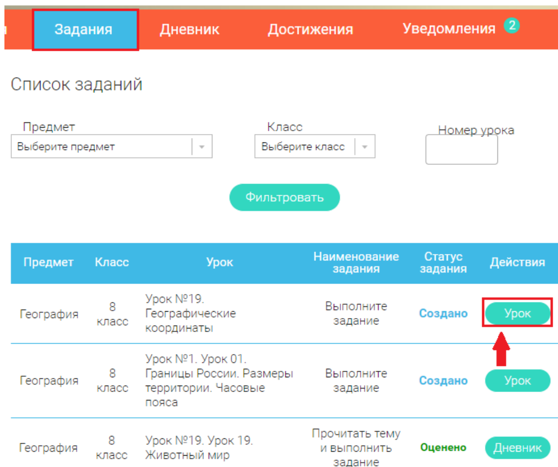
Рисунок 8 – Просмотр заданий
