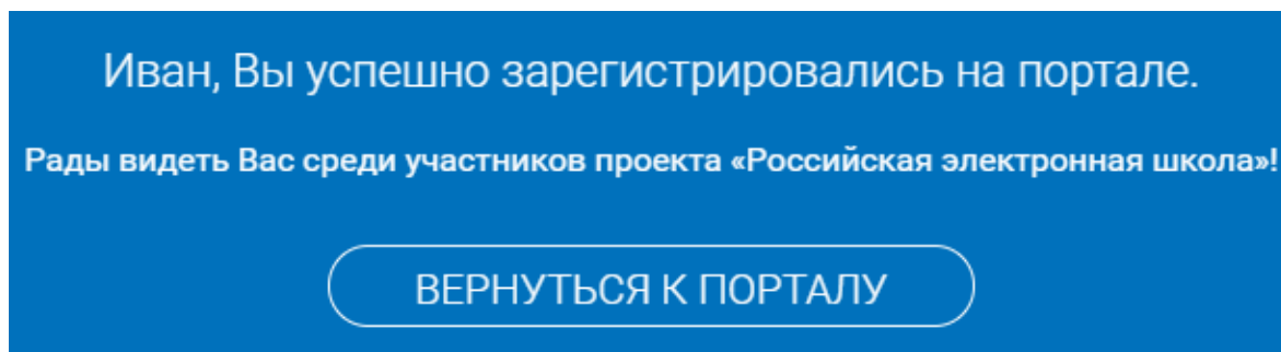
Рисунок 3 – Подтверждение регистрации
